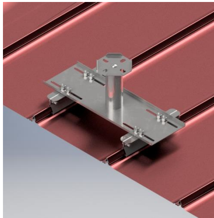
figura 3. Dispositivo GEN 6.0 S FMAC
