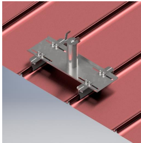
figura 2. Elemento intermedio Tipo C modello GEN 6.0 I FMAC
