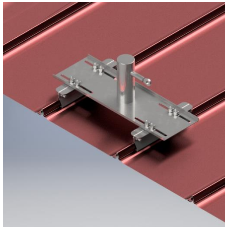
figura 1. Elemento terminale Tipo C modello GEN 6.0 T FMAC
