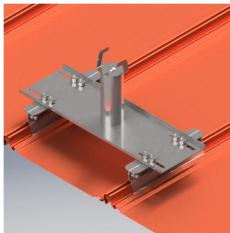
figura 2. Elemento intermedio Tipo C modello GEN 6.0 I FRK
