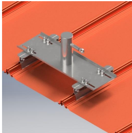
figura 1. Elemento terminale Tipo C modello GEN 6.0 T FRK
