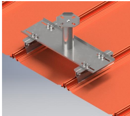
figura 3. Dispositivo GEN 6.0 S FRK
