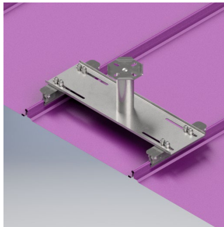
figura 3. Dispositivo GEN 6.0 S FSH
