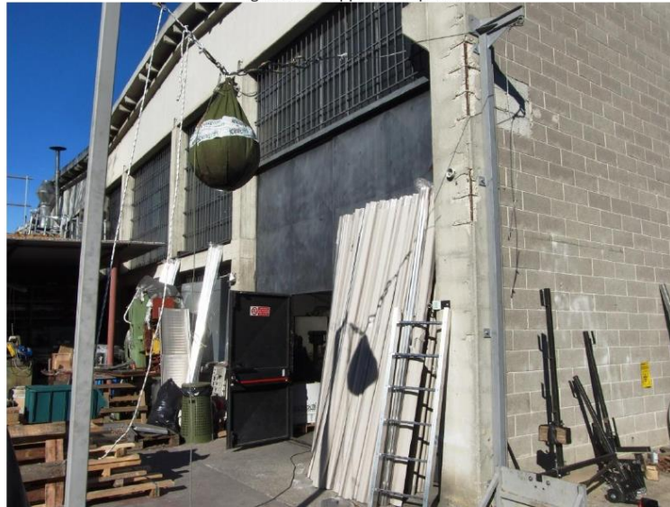
Allestimento prova d'urto - 1100 J
