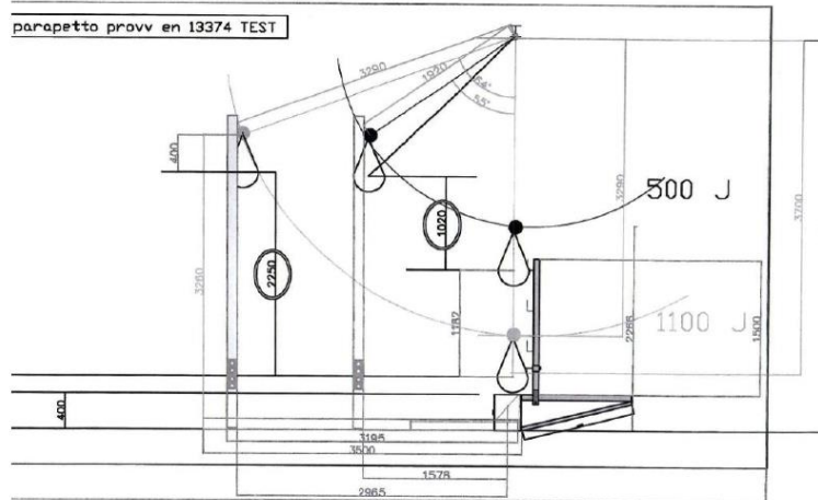
Progettazione apparato di prova
